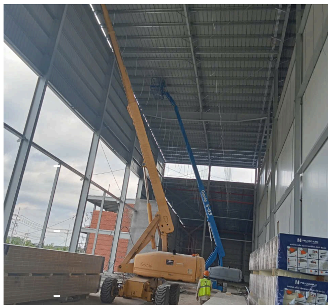
THI CÔNG NHÀ XƯỞNG
